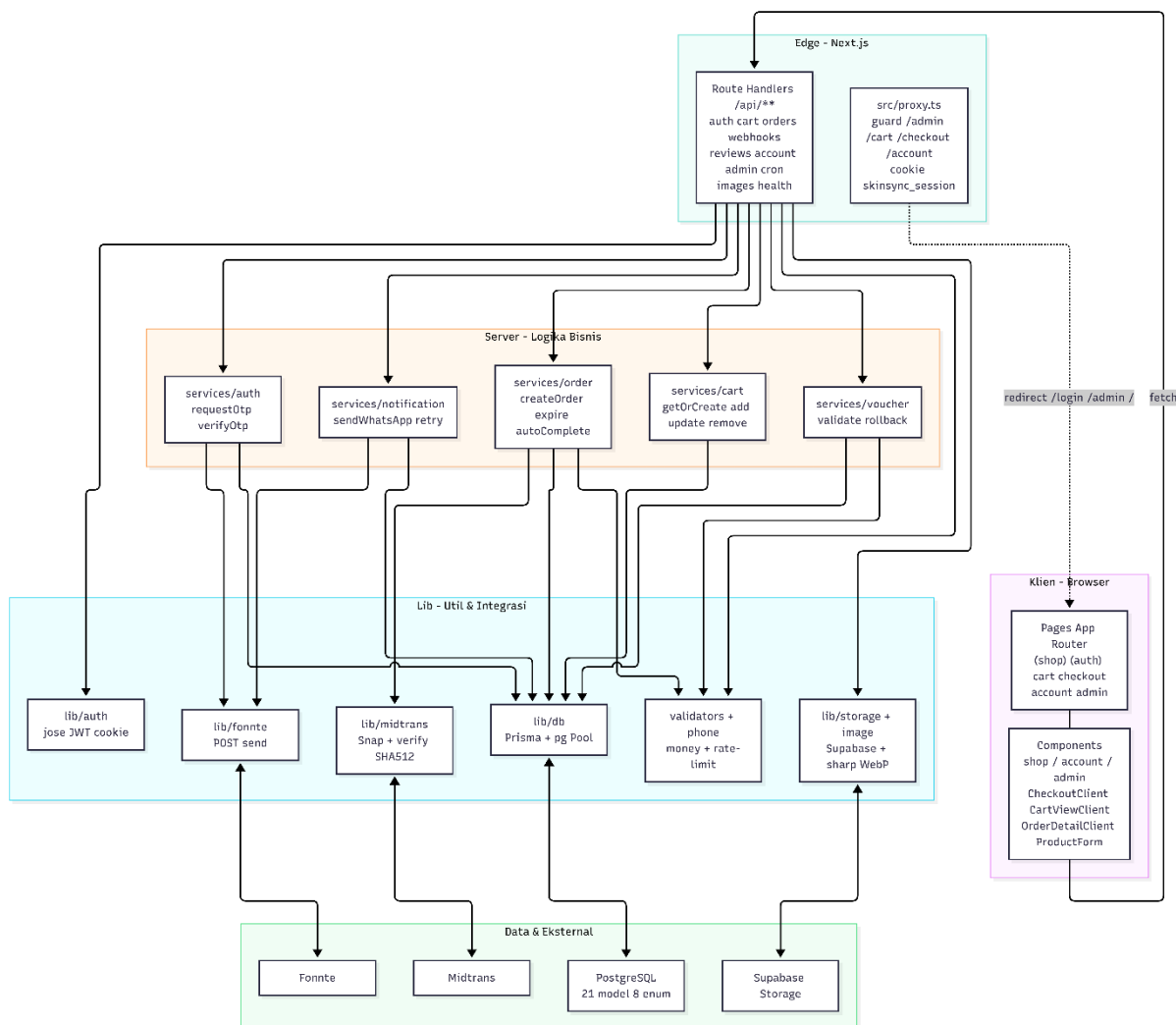
Gambar 5.1 Diagram Arsitektur Sistem
